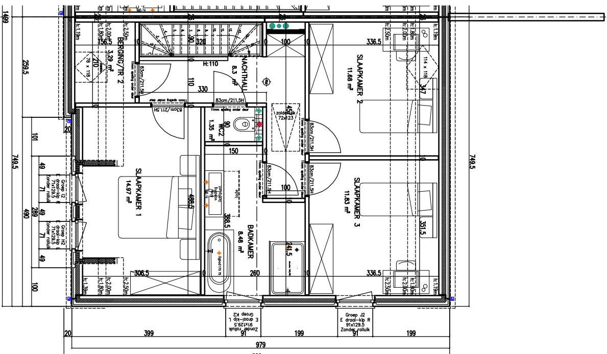
-woning Lot 5- 73.895m² -VERDIEPING-
