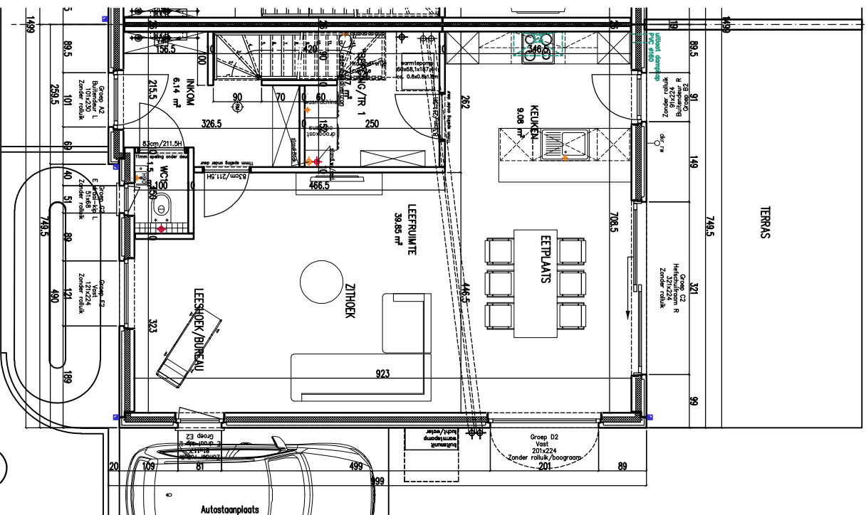
-woning Lot 5- 73.895m² -GRONDPLAN-
