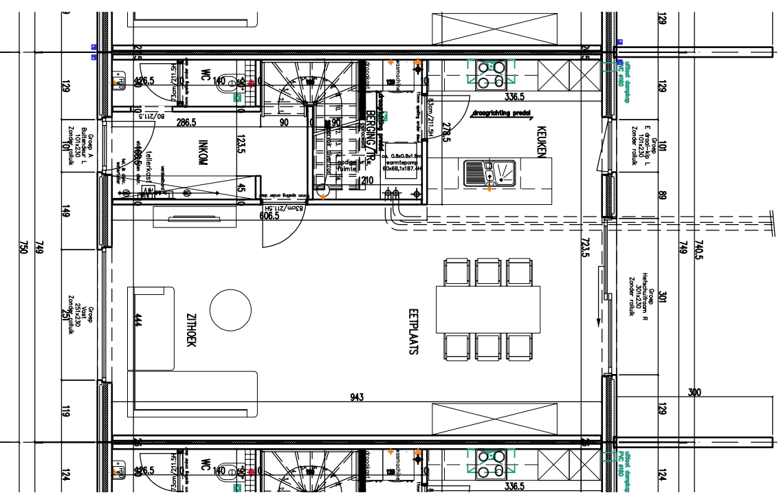
-GELIJKVLOERS- 74,92m 2 PAS 0 Woning L4
