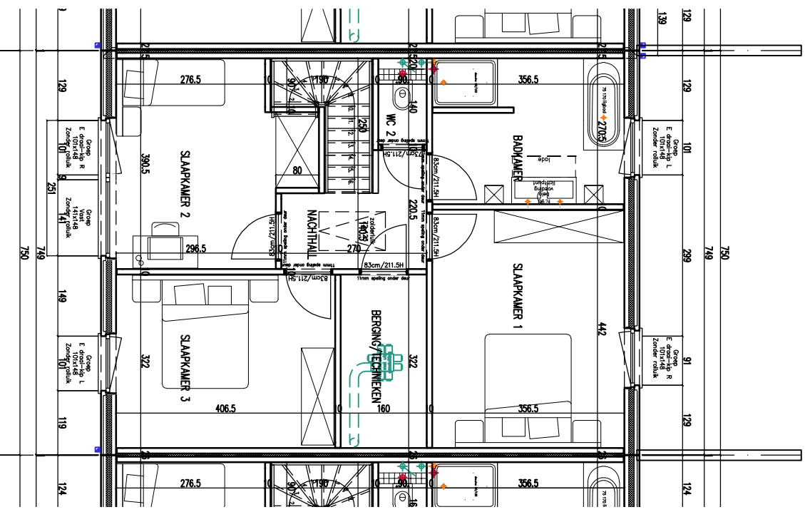
-VERDIEPING+1- 74,92m 2 PAS 291 Woning L4
