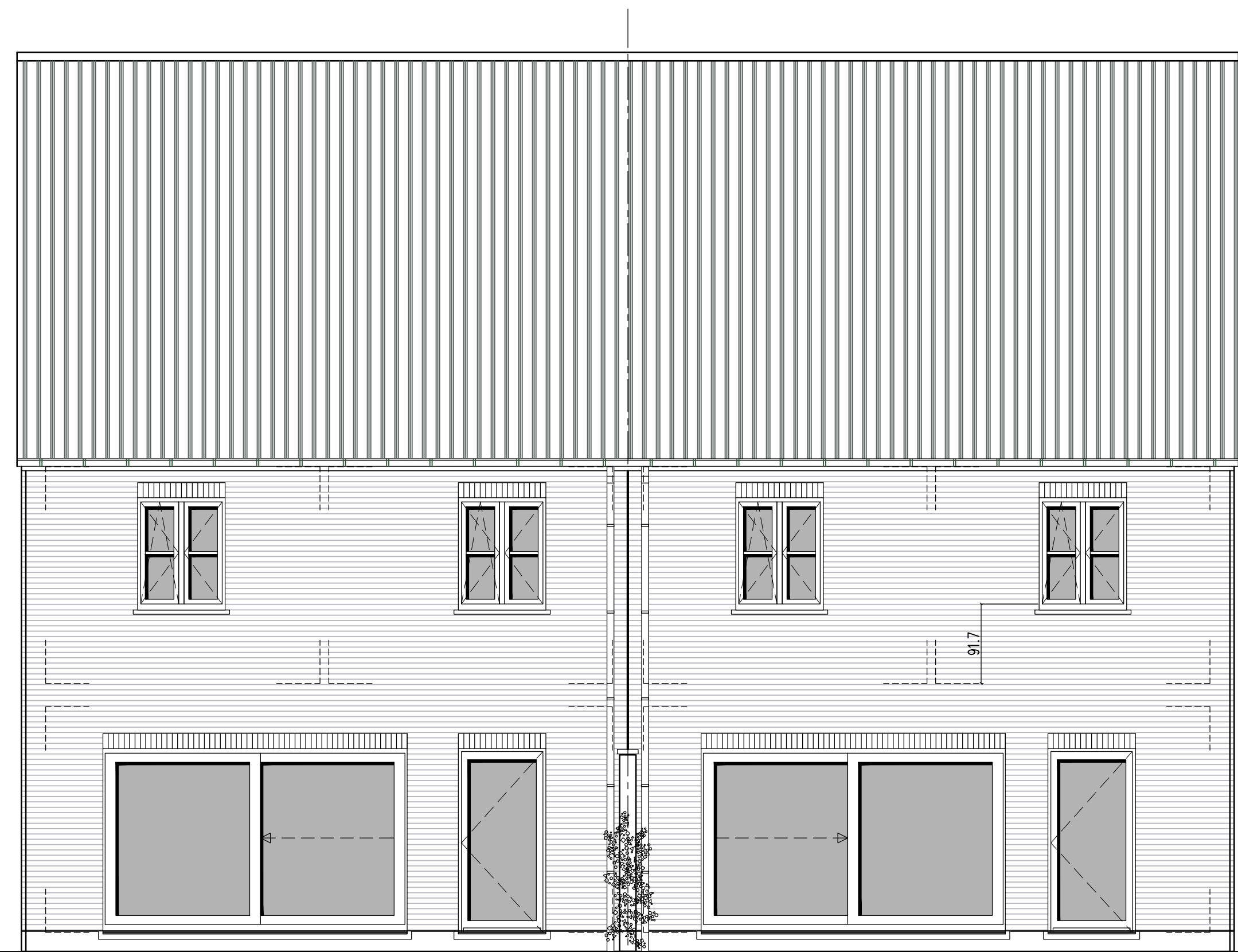
-ACHTERGEVEL- Lot 7
