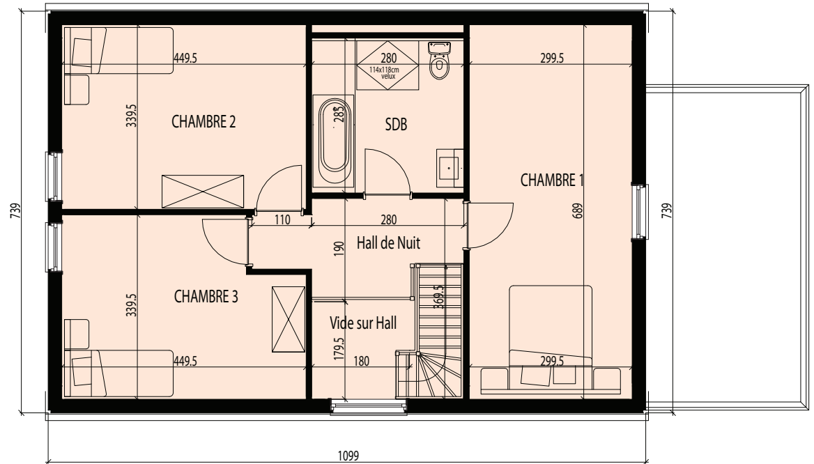
ETAGE - 81m 2
