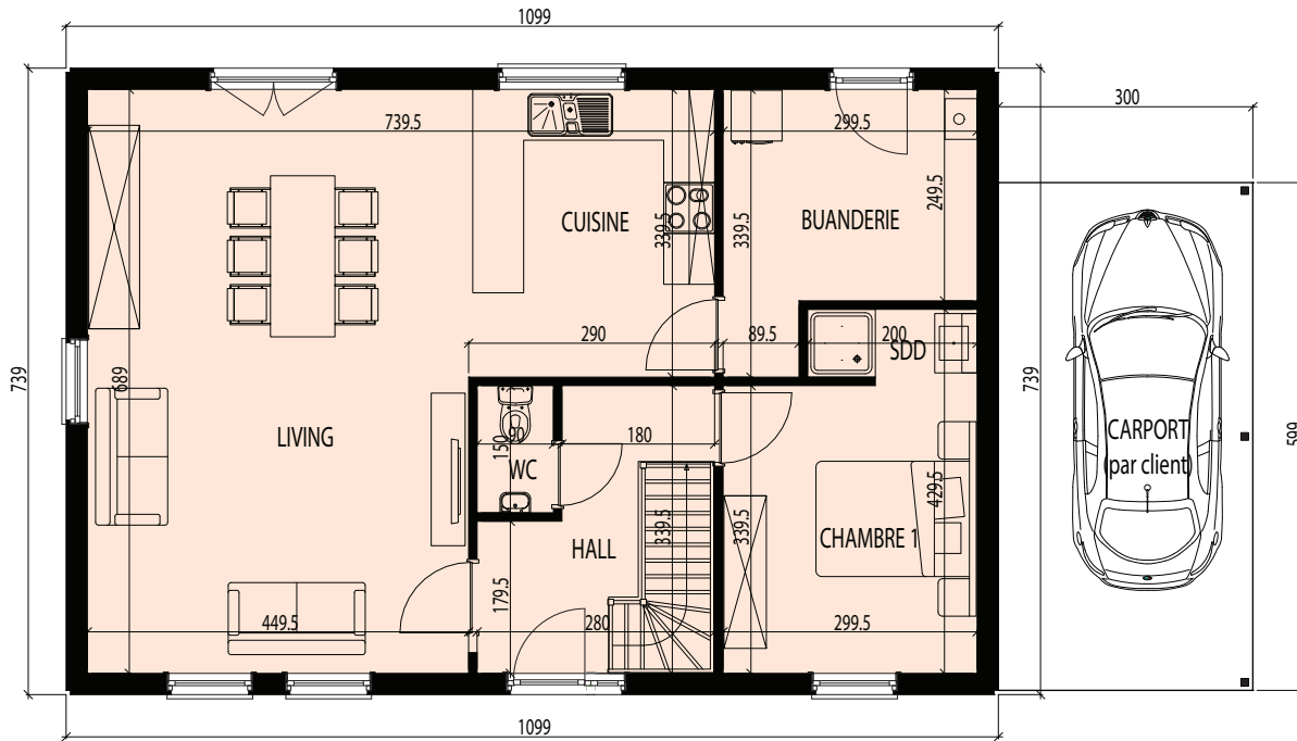
REZ-DE-CHAUSSEE - 81m 2
