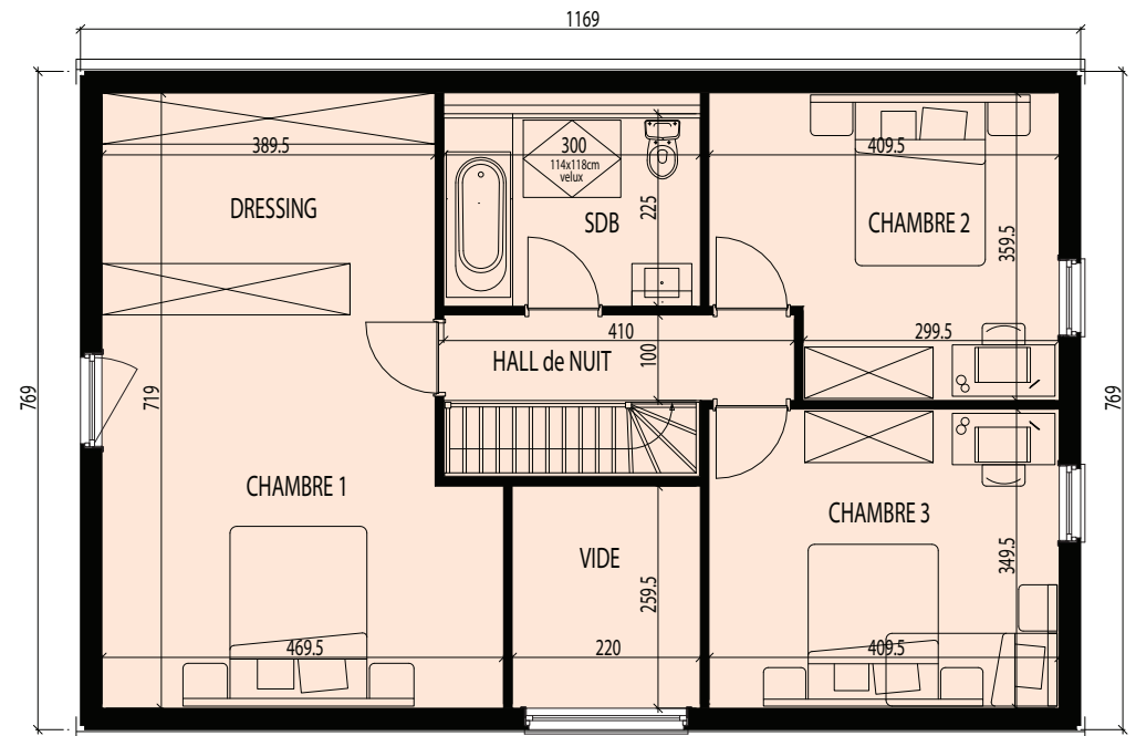
ETAGE - 90m 2
